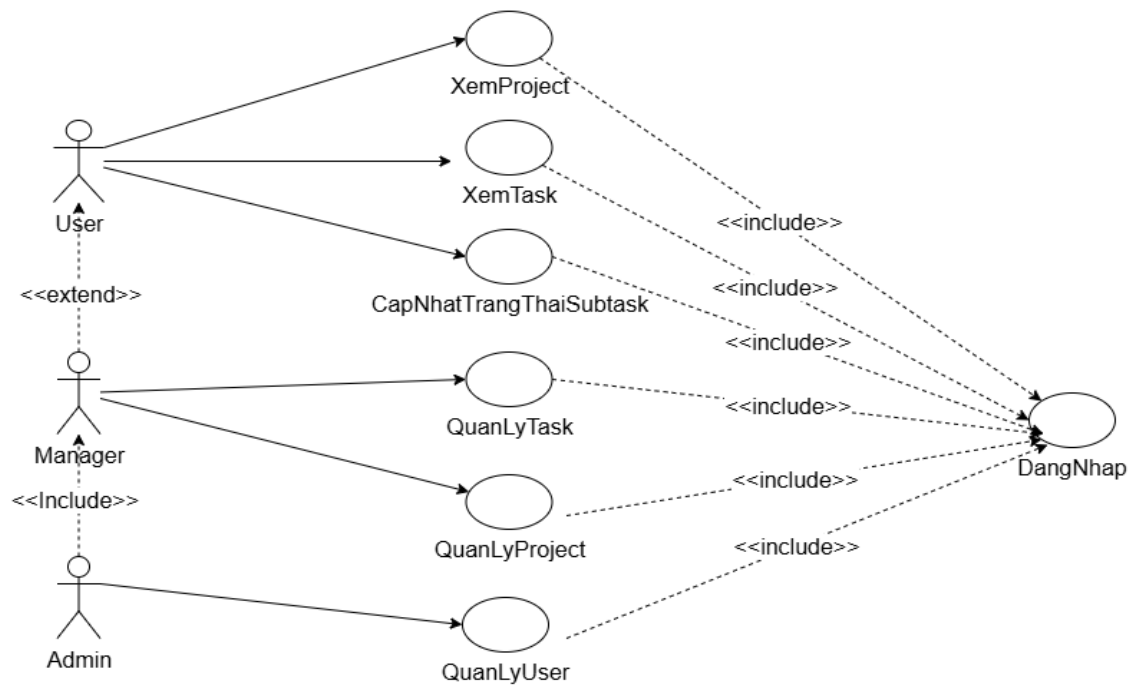
Hình 2.1. Biểu đồ Usecase tổng quát
