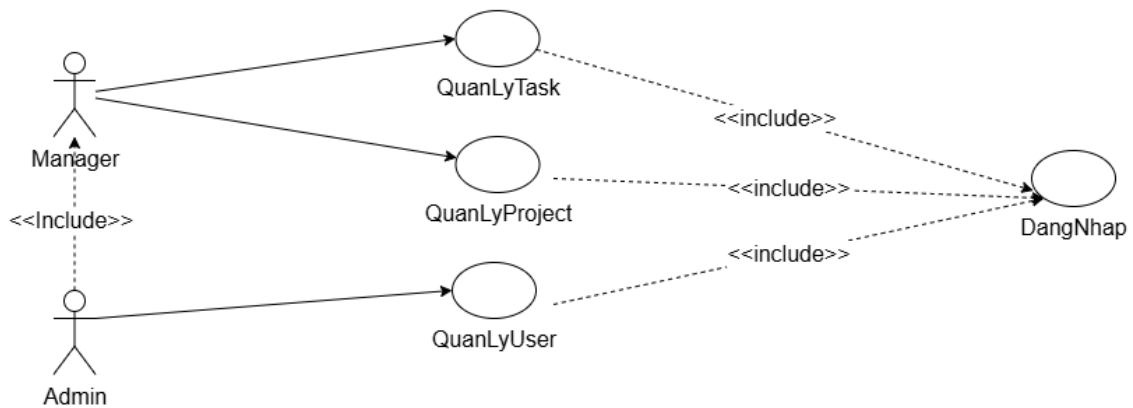
Hình 2.2. Biểu đồ Usecase chính
